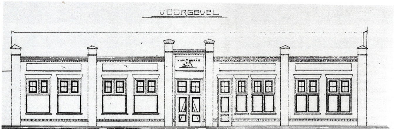
Voorgevel fabrieksgebouw van Mouwerik en Bal aan de Dalweg te Zeist - Bouwtekening 1919
